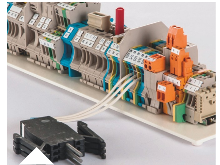
Reihenklemmen enthalten Federn aus Hochleistungslegierungen, wie z. B. Wieland-K55 R800
